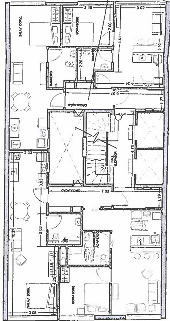
PAVIMENTO TIPO
